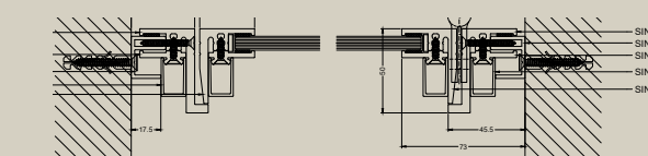
DOOR
