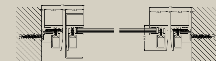
PIVOT DOOR
